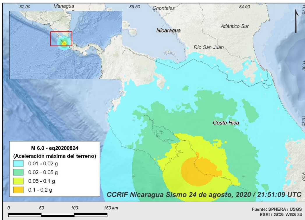
Figura 2 Mapa que muestra la aceleración máxima del terreno originada en Nicaragua por el sismo de magnitud 6.0 del 24 de agosto de 2020 a las 21:51:09 UTC. Fuente: USGS & CCRIF SPHERA .
