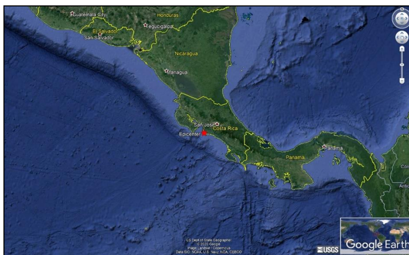
Figura 1 Información del Servicio Geológico de los Estados Unidos (USGS) referente al epicentro del evento sísmico del 24 de agosto de 2020 a las 21:51:09 UTC. Fuente: USGS 1
