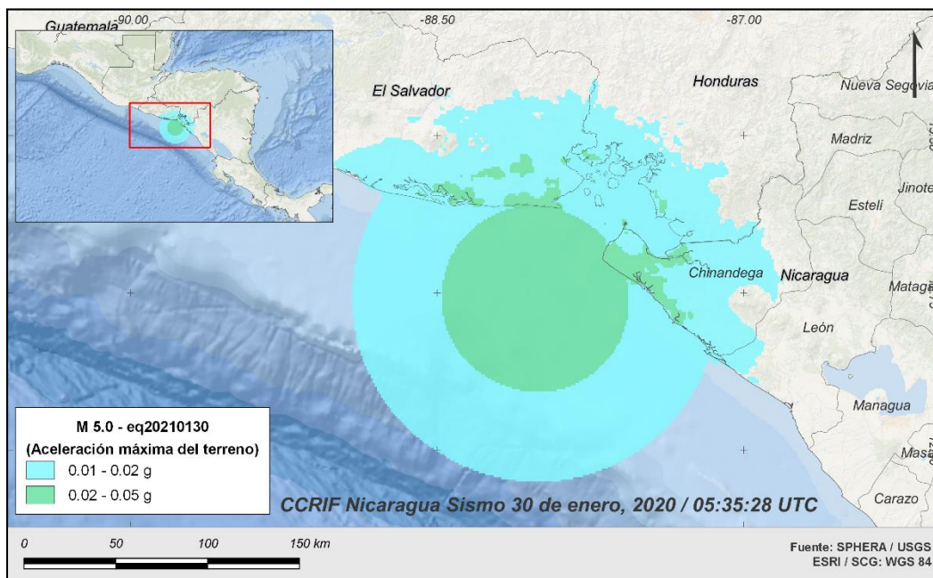
Figura 2 Mapa que muestra la aceleración máxima del terreno originada en Nicaragua por el sismo de magnitud 5.0 del 30 de enero de 2021 a las 05:35:28 UTC. Fuente: USGS & CCRIF SPHERA .
