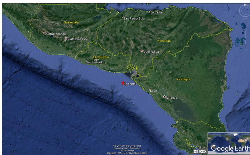
Figura 1 Información del Servicio Geológico de los Estados Unidos (USGS) referente al epicentro del evento sísmico del 30 de enero de 2021 a las 05:35:28 UTC. Fuente: USGS 1
